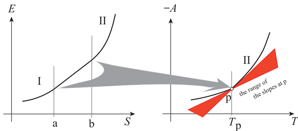
Figure 23.4: ab の間でエントロピーは変化するが温度は一定であるとする、 E のグラフは ab 間では一定の傾きを持つてのっぺりとしてしまう．この部分は Legendre-Fenchel 変換ではその傾きに対応した温度の一点に変換される (そして A が微分不可能になる)．しかし、 p で -A に接する直線群の傾きの範囲 (つまりエントロピーの範囲; 赤い扇形、これは劣微分の図示になっている → C.3 ) は A のグラフからも失われていないので復元できる．もちろん元の点が「矢印」の根元のどこから来たかはわからなくなる．これが T が熱力学座標として採用できない理由である．
