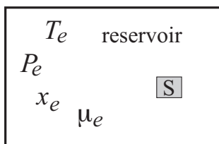
Figure Ex22.1: 系 S は巨大な孤立系の一部であり (全体が巨大なので) 示強変数 T_e, P_e など是一定に保たれていると考えてよい。これらの共役変数 ( S, V , など) は系と残りの部分との間で自由にやりとりできるとする。
