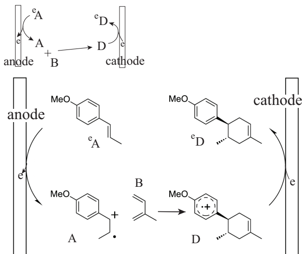
Figure Ex26.1: 電解合成 {}^e\text{A} + \text{B} \longrightarrow {}^e\text{D} の例. Y. Imada, Y. Okada and K. Chiba, Investigating radical cation chain processes in the electrocatalytic Diels-Alder reaction, Beilstein J. Org. Chem., 14 , 642 (2018) の図 1 に基づく. A: trans -アネトール, B: イソプレン, そして D が Diels-Alder 付加物. 電位差 1 V が使われた.
